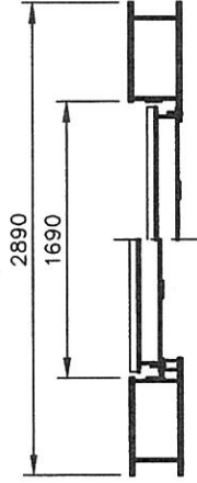
DOORSNEDE A-A SCHAAL 1:25
